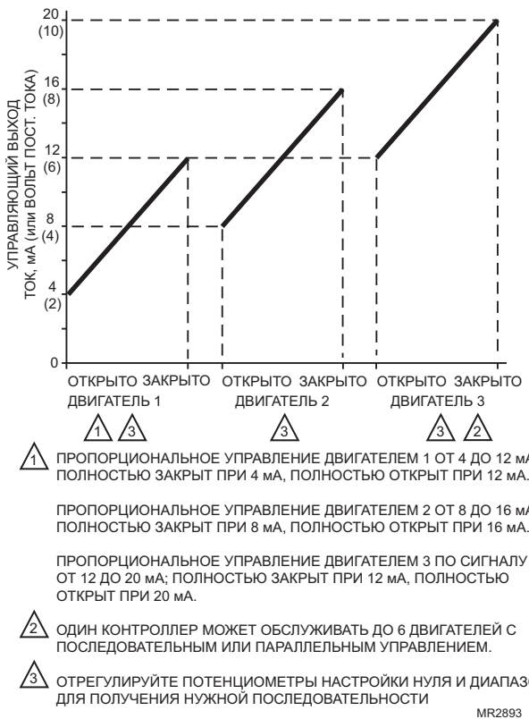
Рис. 11. Последовательная схема работы двигателей.
