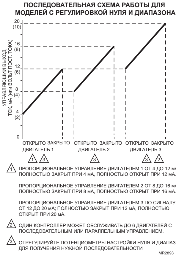
Рис. 11. Последовательная схема работы двигателей.
