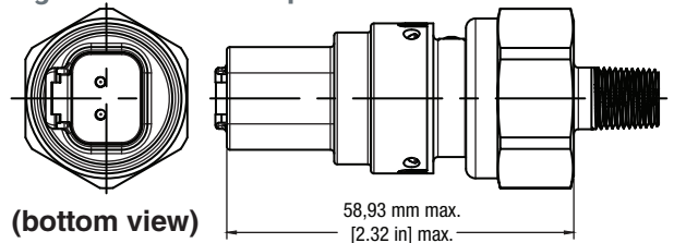
Figure 23. Deutsch 2-pin
