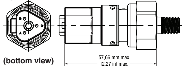
Figure 22. Deutsch 3-pin
