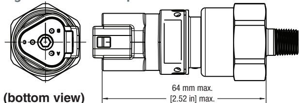
Figure 15. Deutsch 3-pin
