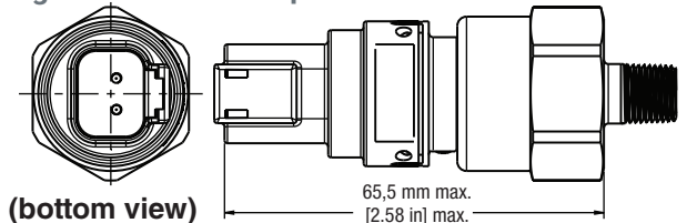
Figure 16. Deutsch 2-pin
