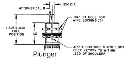
400EN actuators
