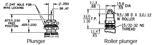
400EN actuators
