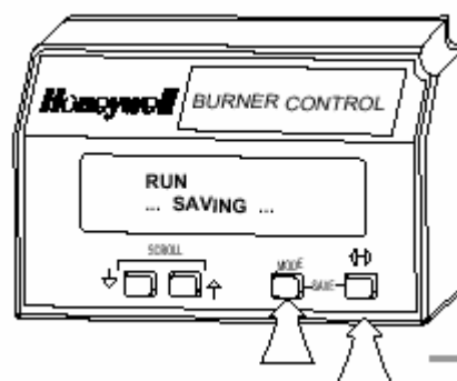
Рис. 21. Функция SAVE.
