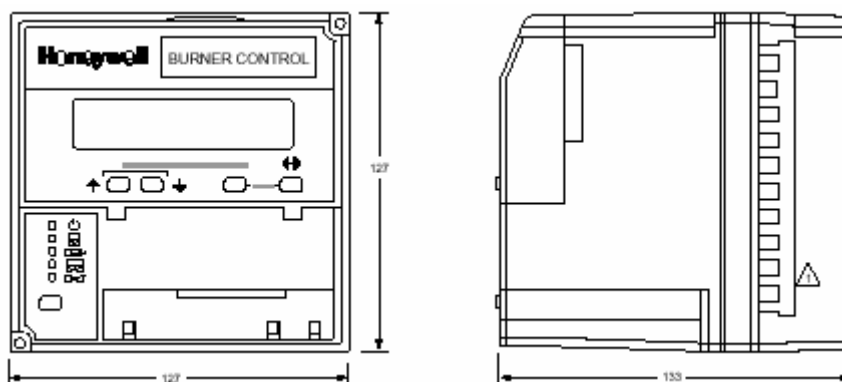
Рис. 1. Размеры Модуля реле и основания Q7800A, в миллиметрах.
