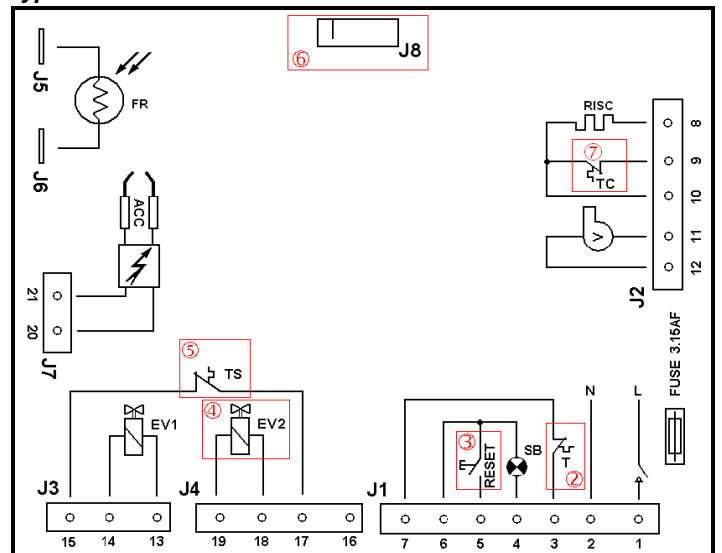
Type DTMN320
