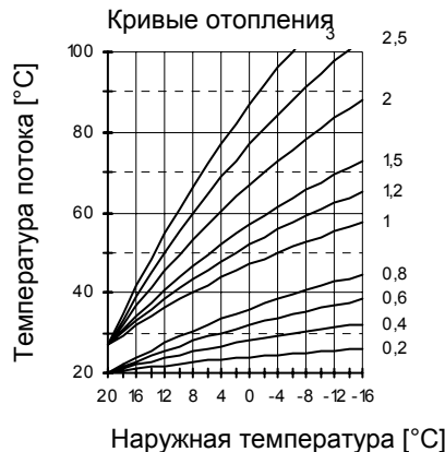
Кривая отопления
