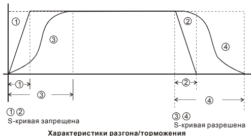
Характеристики разгона/торможения
