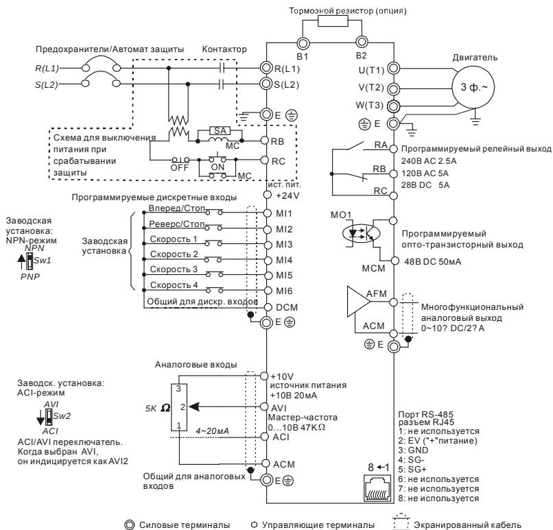
Рисунок 5. Схема для моделей VFD002E11T/21T, VFD004E11A/21T, VFD007E21T.
