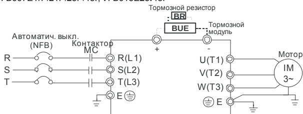
Схема 2 (для типоразмеров В): VFD007E11A, VFD015E21A, VFD022E21A/23A/43A VFD037E23A/43A, VFD007E11C, VFD015E21C, VFD022E21C/23C/43C, VFD037E23C/43C (для типоразмера С): VFD055E23A/43A, VFD075E23A/43A, VFD110E43A, VFD055E23C/43C, VFD075E23C/43C, VFD110E43C (для типоразмера D): VFD150E23A/23C, VFD150E43A/43C, VFD185E43A/43C, VFD220E43A/43C
