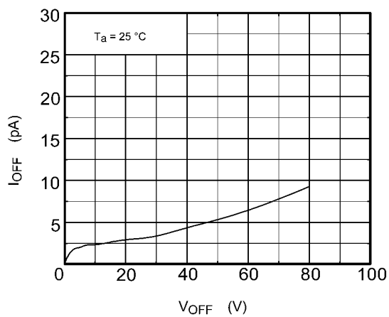
Fig. 12.9 I_{OFF} - V_{OFF}
