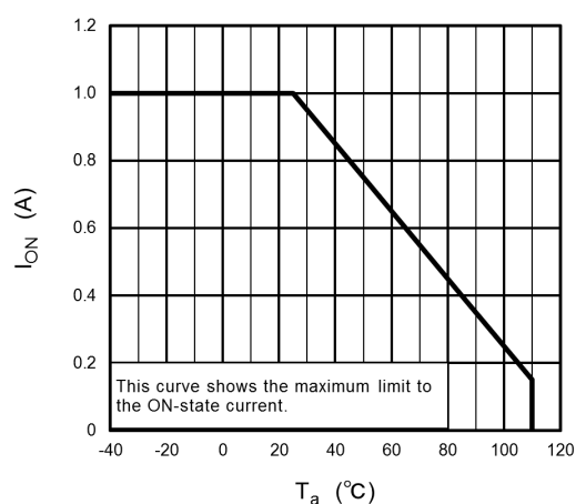
Fig. 12.1 I_{ON} - T_a
