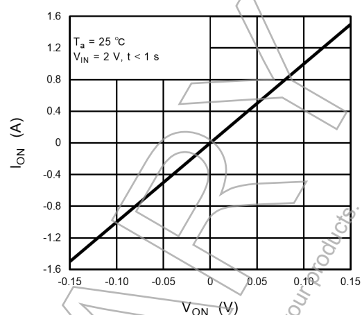
Fig. 12.2 I_{ON} - V_{ON}
