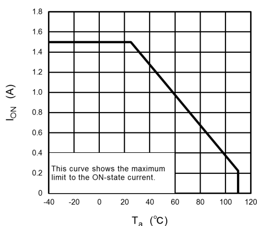
Fig. 12.1 I_{ON} - T_a
