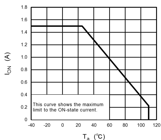
Fig. 12.2 I_{ON} - T_a
