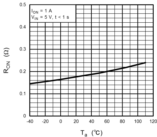
Fig. 12.3 R_{ON} - T_a
