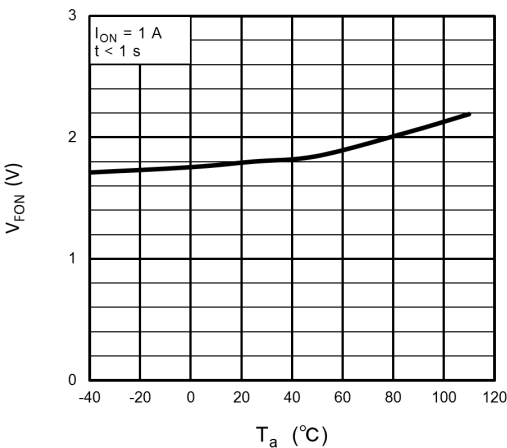
Fig. 12.4 V_{FON} - T_a
