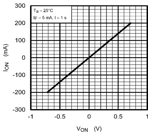
Fig. 12.1.4 I_{ON} - V_{ON}
