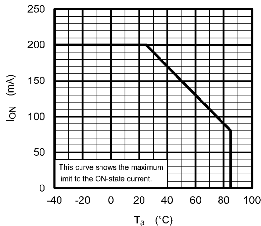
Fig. 12.1.2 I_{ON} - T_a
