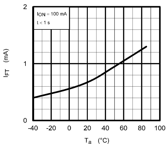
Fig. 12.1.6 I_{FT} - T_a
