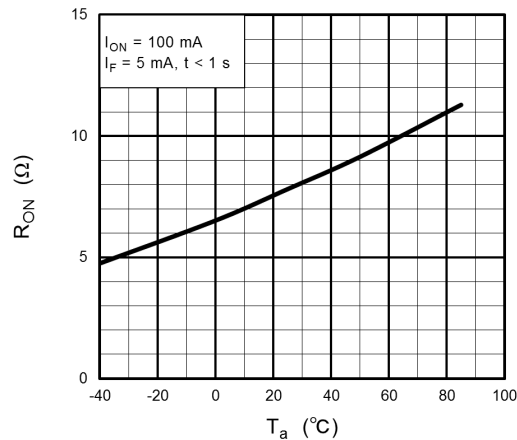
Fig. 12.1.5 R_{ON} - T_a
