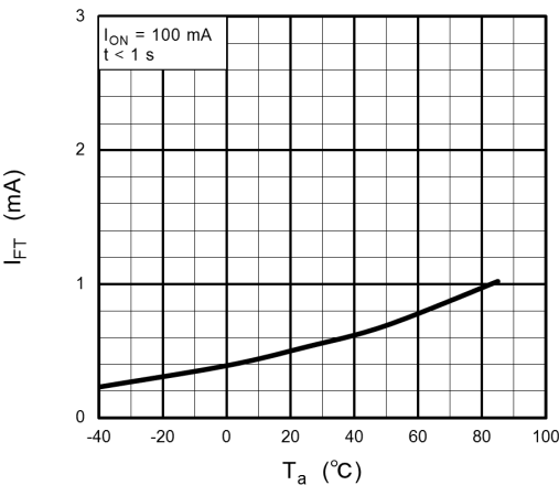
Fig. 12.1.6 I_{FT} - T_a
