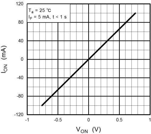
Fig. 12.1.4 I_{ON} - V_{ON}
