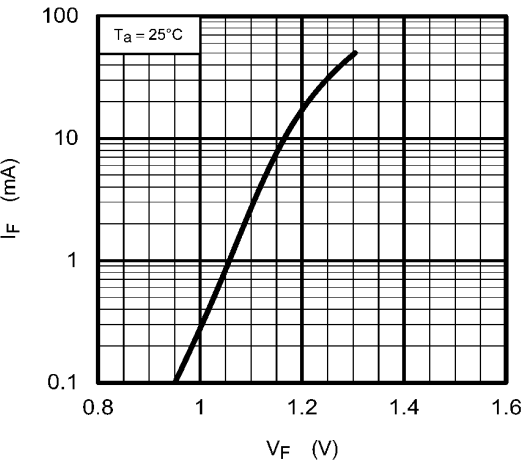
Fig. 12.1.3 I_F - V_F
