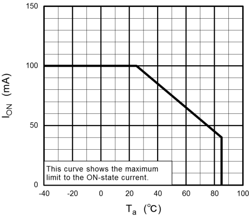
Fig. 12.1.2 I_{ON} - T_a
