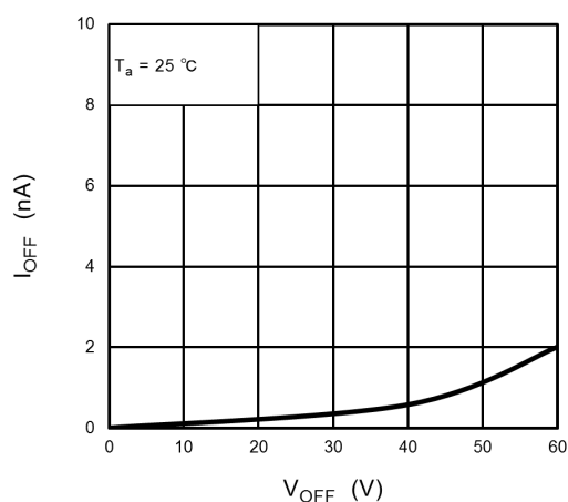
Fig. 14.1.10 I_{OFF} - V_{OFF}
