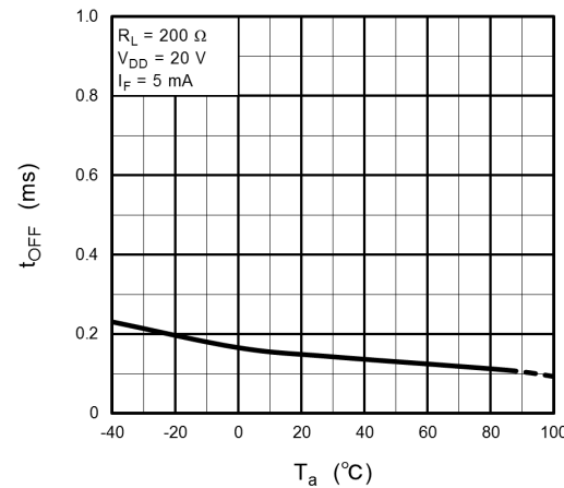
Fig. 12.1.8 t_{OFF} - T_a
