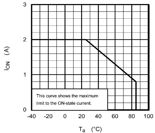
Fig. 16.2 I_{ON} - T_a
