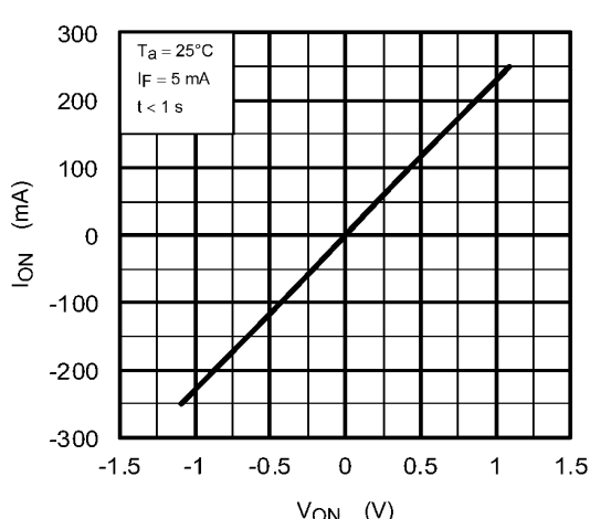
Fig. 16.4 I_{ON} - V_{ON}
