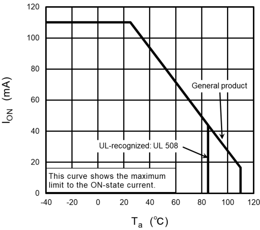
Fig. 14.1.2 I_{ON} - T_a
