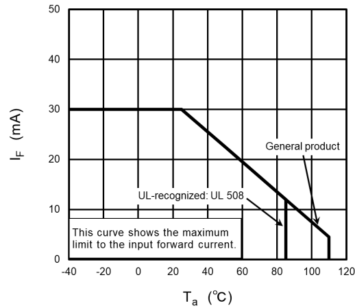
Fig. 14.1.1 I_F - T_a
