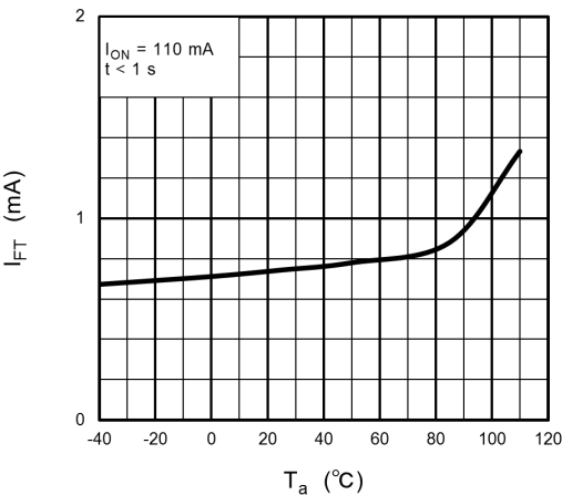
Fig. 14.1.6 I_{FT} - T_a
