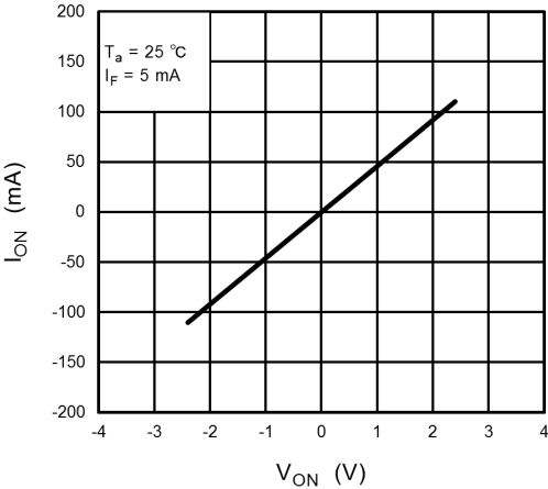
Fig. 14.1.4 I_{ON} - V_{ON}
