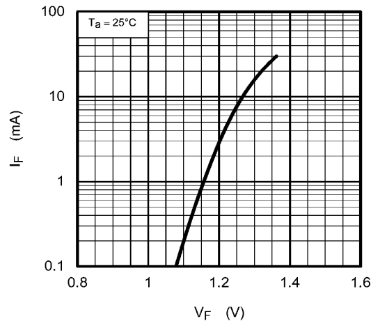
Fig. 14.1.3 I_F - V_F
