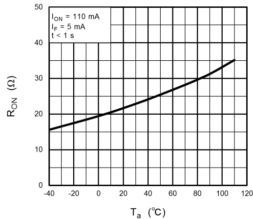
Fig. 14.1.5 R_{ON} - T_a
