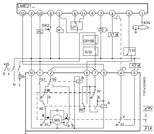
SQN3...121.../2-ступенчатое управление
