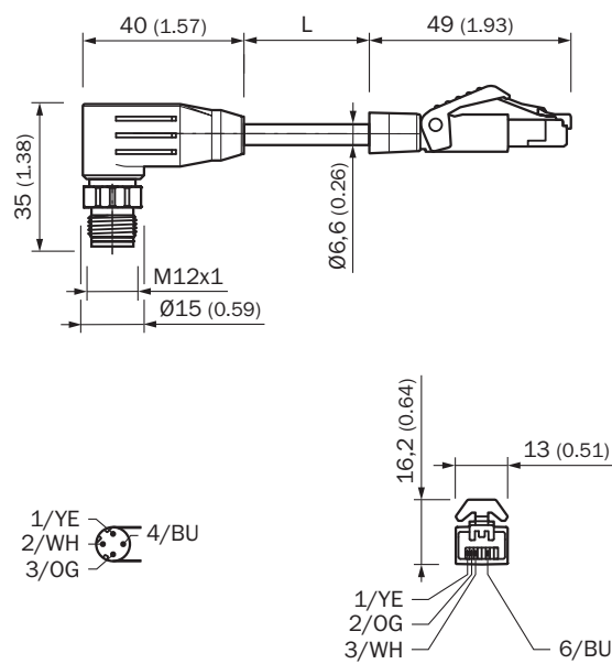
Габаритный чертеж (Размеры, мм)
