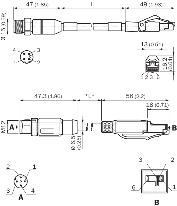
Габаритный чертеж (Размеры, мм)
