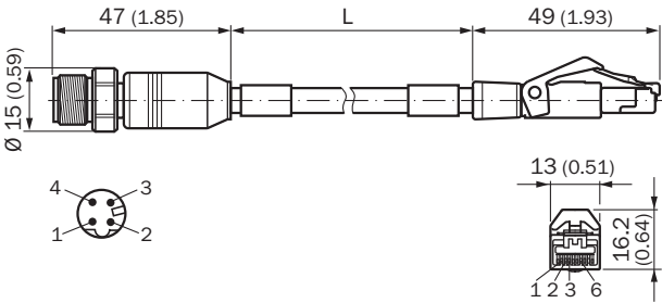
Габаритный чертеж (Размеры, мм)
