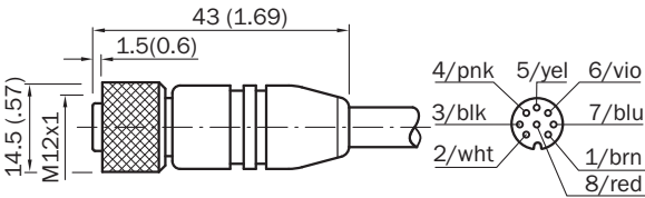
Габаритный чертеж (Размеры, мм)
