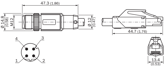
Габаритный чертеж (Размеры, мм)
