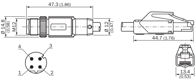
Габаритный чертеж (Размеры, мм)
