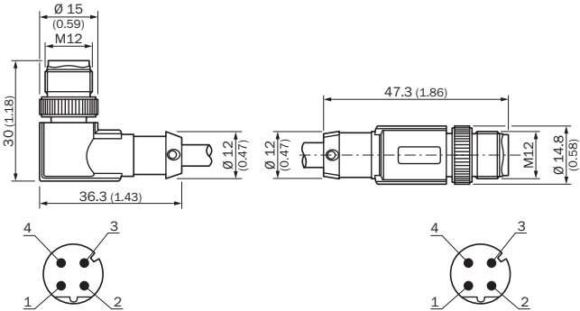
Габаритный чертеж (Размеры, мм)
