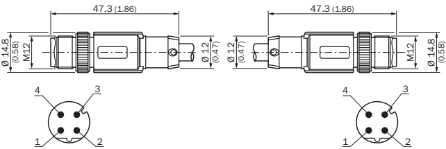
Габаритный чертеж (Размеры, мм)
