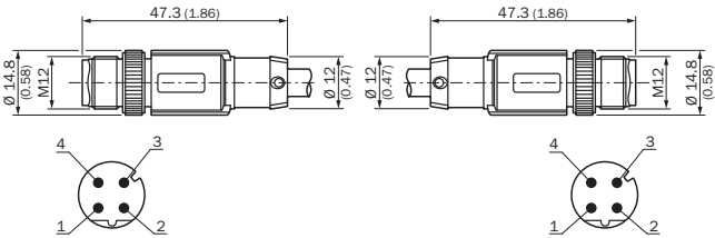
Габаритный чертеж (Размеры, мм)
