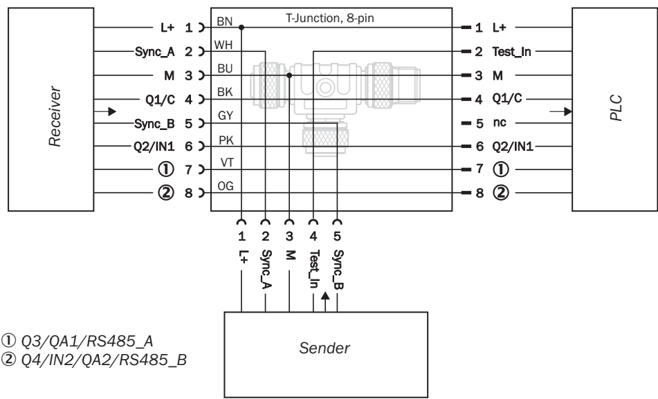
Схема подключения тройника
