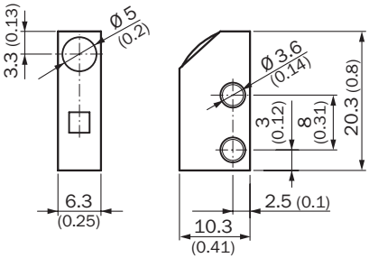
Габаритный чертёж (Размеры, мм)
