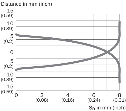
Кривая срабатывания
