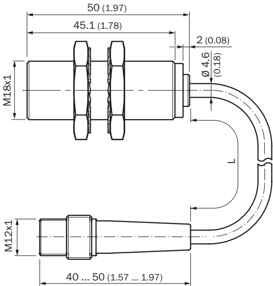
IMB18 стандарт, штекер M12, вровень с плоскостью
