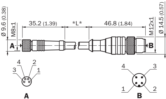
Габаритный чертеж (Размеры, мм)
