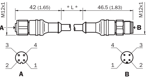
Габаритный чертеж (Размеры, мм)
