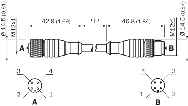
Габаритный чертеж (Размеры, мм)
