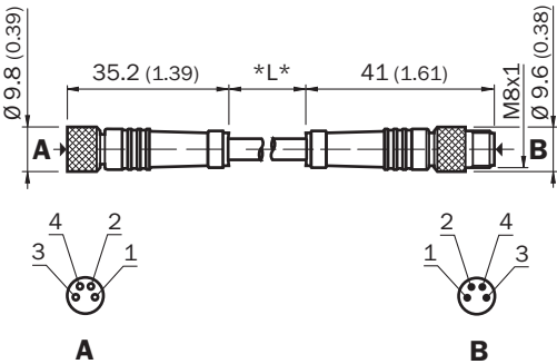
Габаритный чертеж (Размеры, мм)
