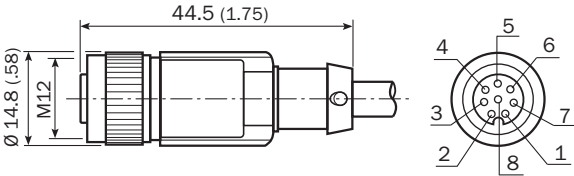
Габаритный чертеж (Размеры, мм)
