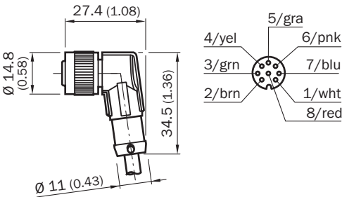
Габаритный чертеж (Размеры, мм)
