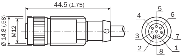
Габаритный чертеж (Размеры, мм)
