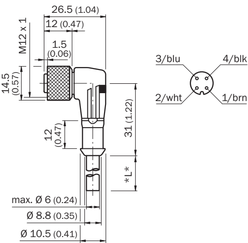
Габаритный чертеж (Размеры, мм)
