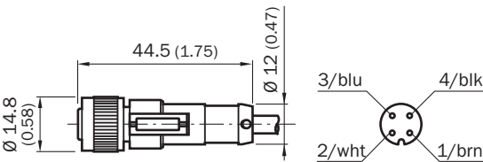
Габаритный чертеж (Размеры, мм)
