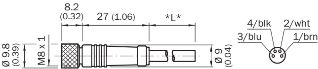
Габаритный чертеж (Размеры, мм)
