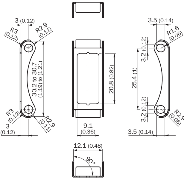
Габаритный чертеж (Размеры, мм)
