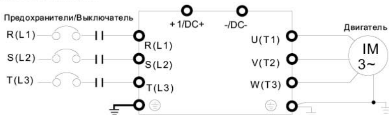
Рисунок 2. Типоразмер D
