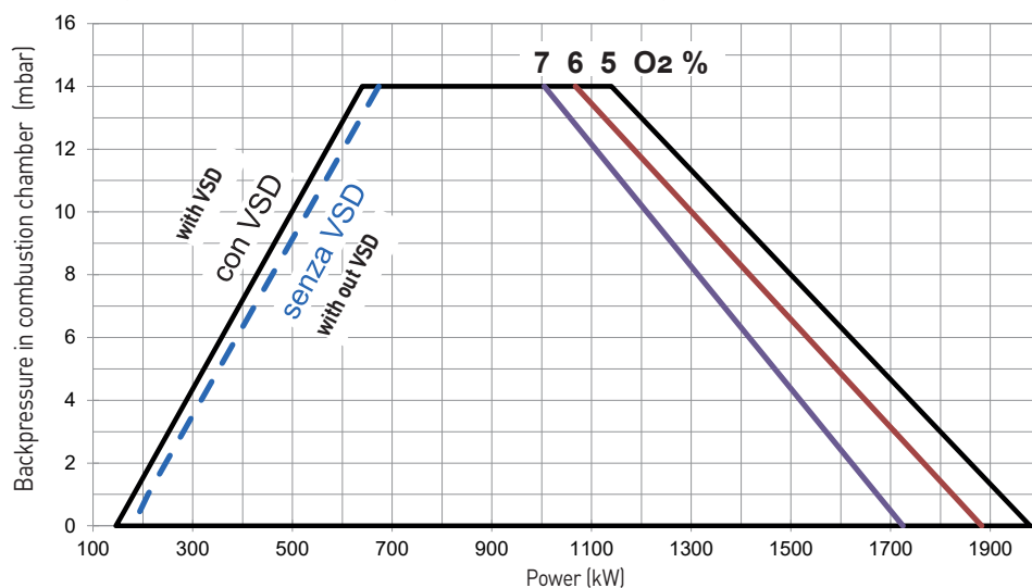
G200N PR-MD
