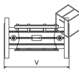
DN65 - DN80
