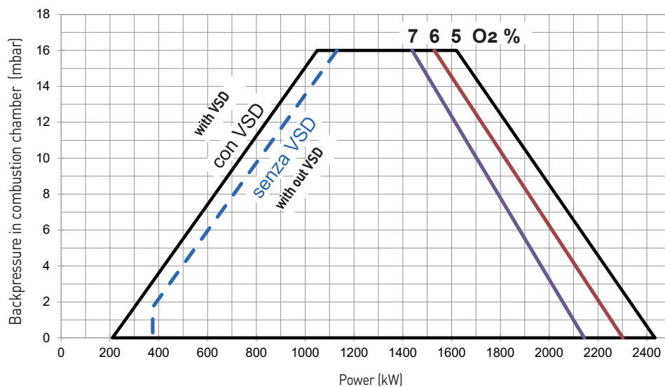
G240N PR-MD
