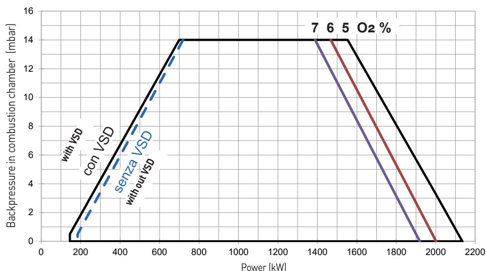
G215N PR-MD
