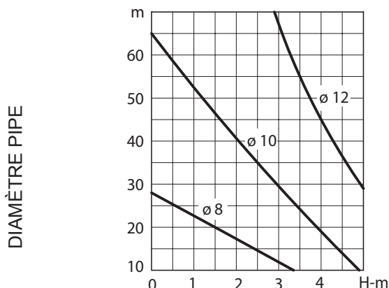
INSTALLATION EN ASPIRATION
