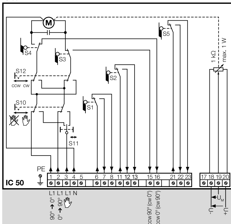
Схема электроподключения IC 50
