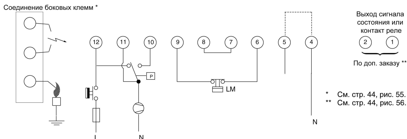
Рис. 53. Схема соединений регуляторов розжига S4565RV и TV с дополнительной предварительной продувкой
