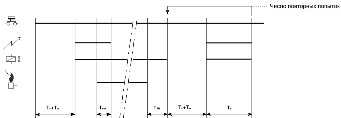
Рис. 59. Диаграмма синхронизации регуляторов розжига S4565PV
